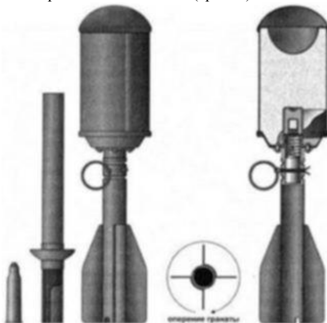
Противотанковая граната ВКГ-42 (ВПГ-42). Слева направо: холостой патрон калибра 7,62x53 мм, ствольная насадка (мортирка) из комплекта гранаты, кумулятивная граната.
