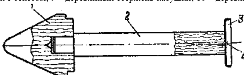
Катушка гранаты: 1 – деревянная головка; 2 – деревянный стержень; 3 – металлическая шайба; 4 – гвоздь.
