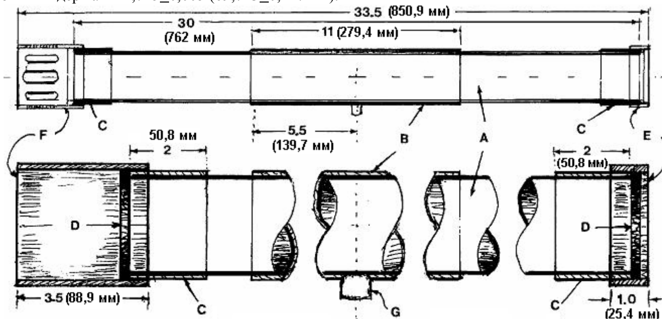
Рис. 3. Часть первая – Сборка пусковой трубы.
