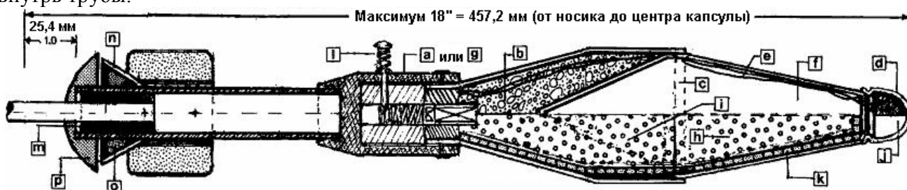
Рис. 8 – Преобразование гранаты М-31. Верхняя половина – противотанковая кумулятивная версия, нижняя половина – противопехотная версия:
