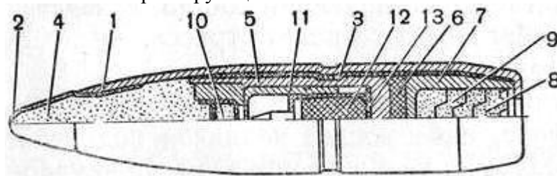
Зажигательная пуля ЗП.
