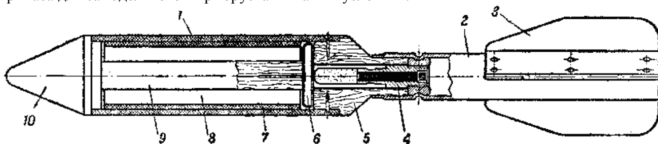
Граната ВАГ-42 в разрезе: 1 – корпус гранаты; 2 – стабилизатор; 3 – перья стабилизатора; 4 – запал; 5 – деревянный поддон; 6 – металлическая шайба; 7 – картонные вкладыши; 8 – место для листовок с текстом; 9 – деревянный стержень катушки; 10 – деревянная головка.
