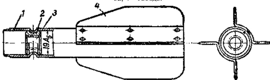
Стабилизатор гранаты: 1 – трубка; 2 – втулка; 3 – навинтованное отверстие для ввинчивания запала; 4 – перья (лопасти) стабилизатора.
